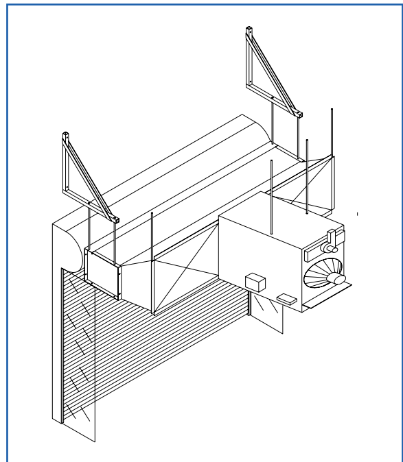
Roll-Up Canister Door
