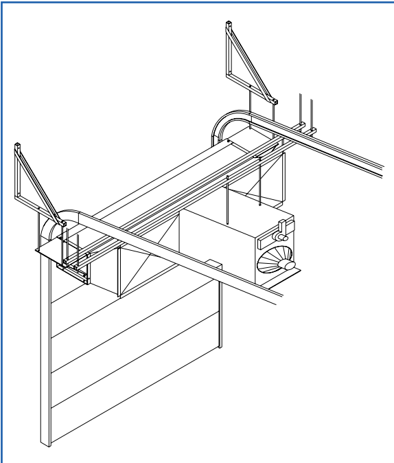
Garage Style Door
